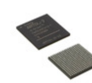
XC7A75T-2CSG324I AMD IC FPGA 210 I/O 324CSBGA
