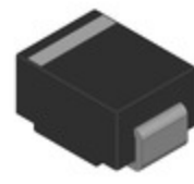
1SMB5947BT3G onsemi DIODE ZENER 82V 3W SMB
