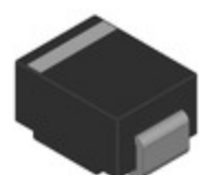
1SMB5942BT3 onsemi DIODE ZENER 51V 3W SMB
