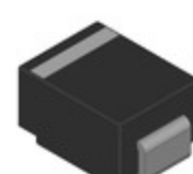
1SMB5918BT3G onsemi DIODE ZENER 5.1V 3W SMB
