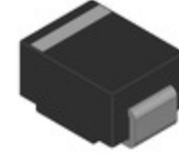
1SMB5938BT3 onsemi DIODE ZENER 36V 3W SMB
