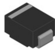
1SMB5945BT3G onsemi DIODE ZENER 68V 3W SMB
