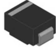
1SMB5942BT3G onsemi DIODE ZENER 51V 3W SMB
