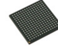
XC6SLX4-2CSG225C AMD IC FPGA 132 I/O 225CSBGA
